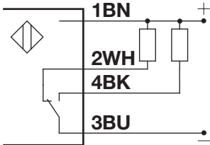
Fig. 2 NPN
