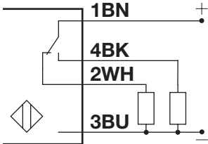
Fig. 3 PNP
