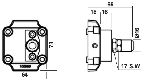
D.B.V Niederdruck (regelbares) interner Rücklauf
