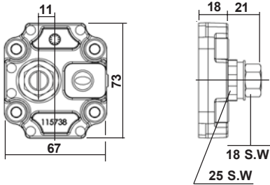
einstellbares D.B.V Hochdruck (fest eingestellt) interner Rücklauf
