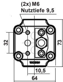
D.B.V Niederdruck (regelbares) externer Rücklauf
