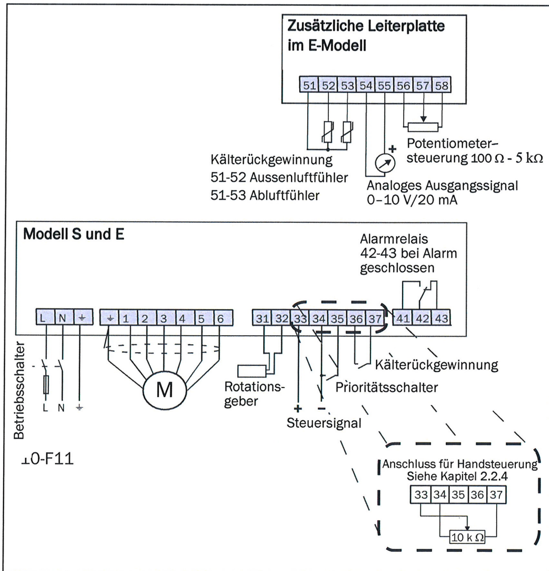
Fig. 6 Anschlussplan
